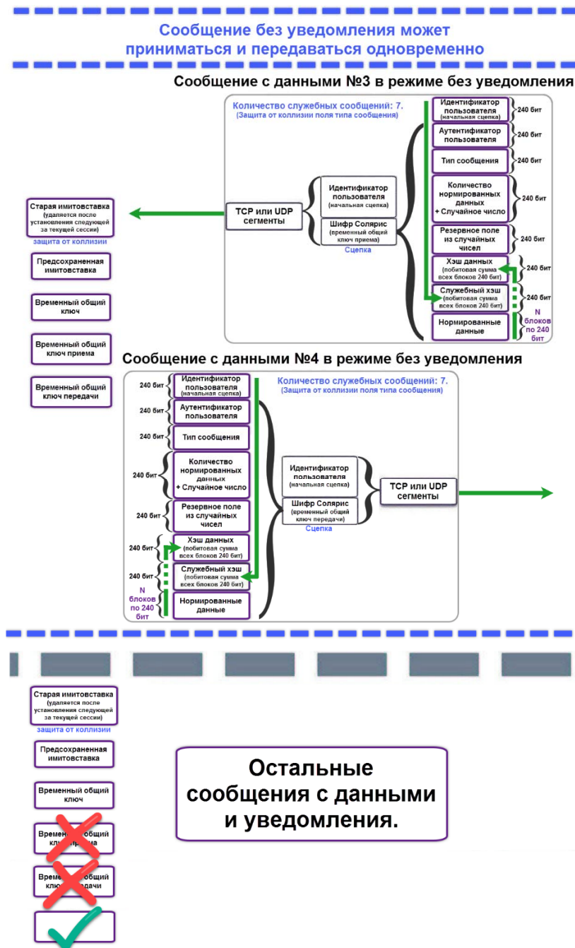
Рис. 6. Схема работы протокола (часть 5)
